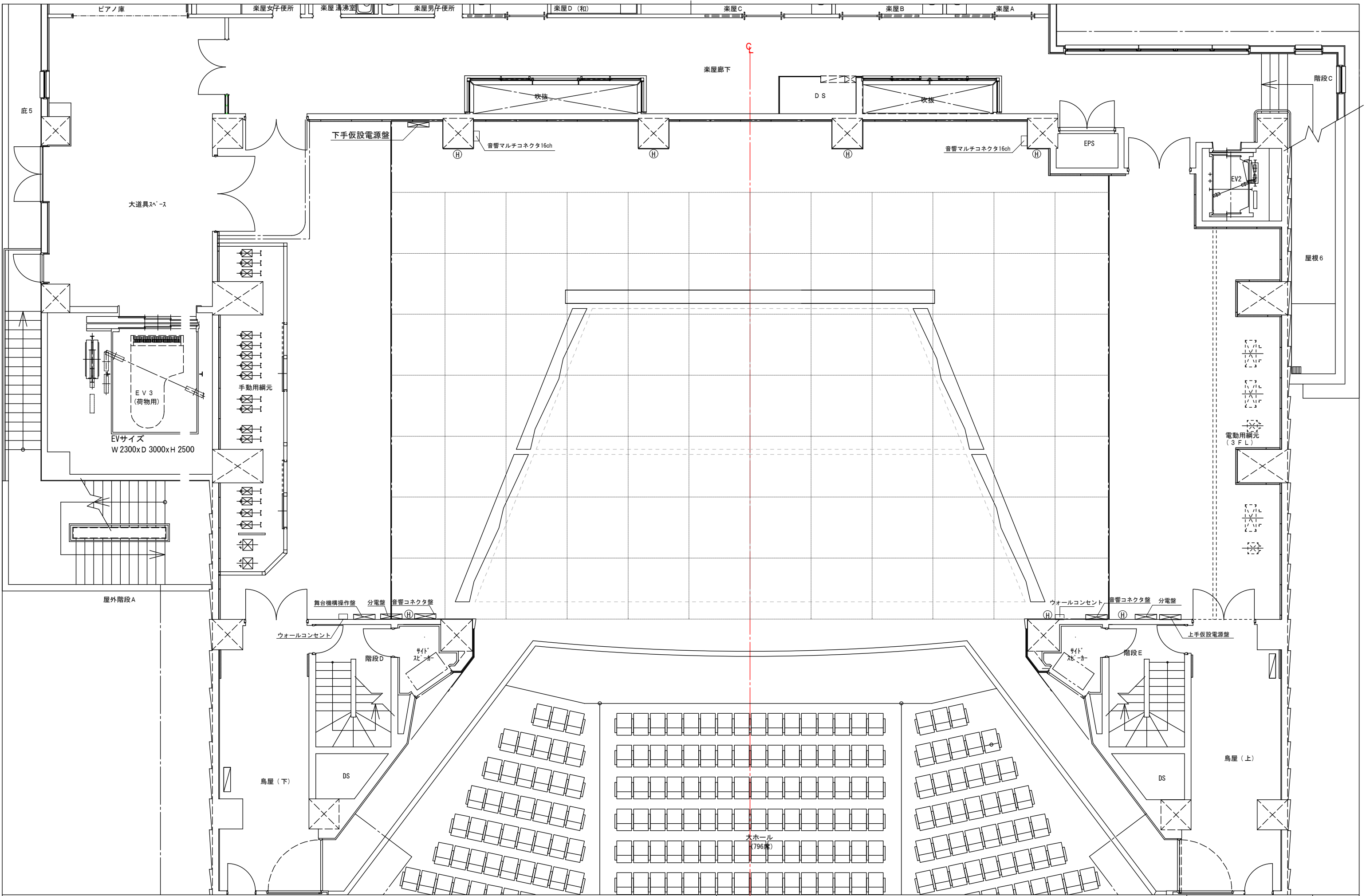
おりなす八女 ハーモニーホール 平面図 (反響板) 縮尺 1/100 (A-3)
