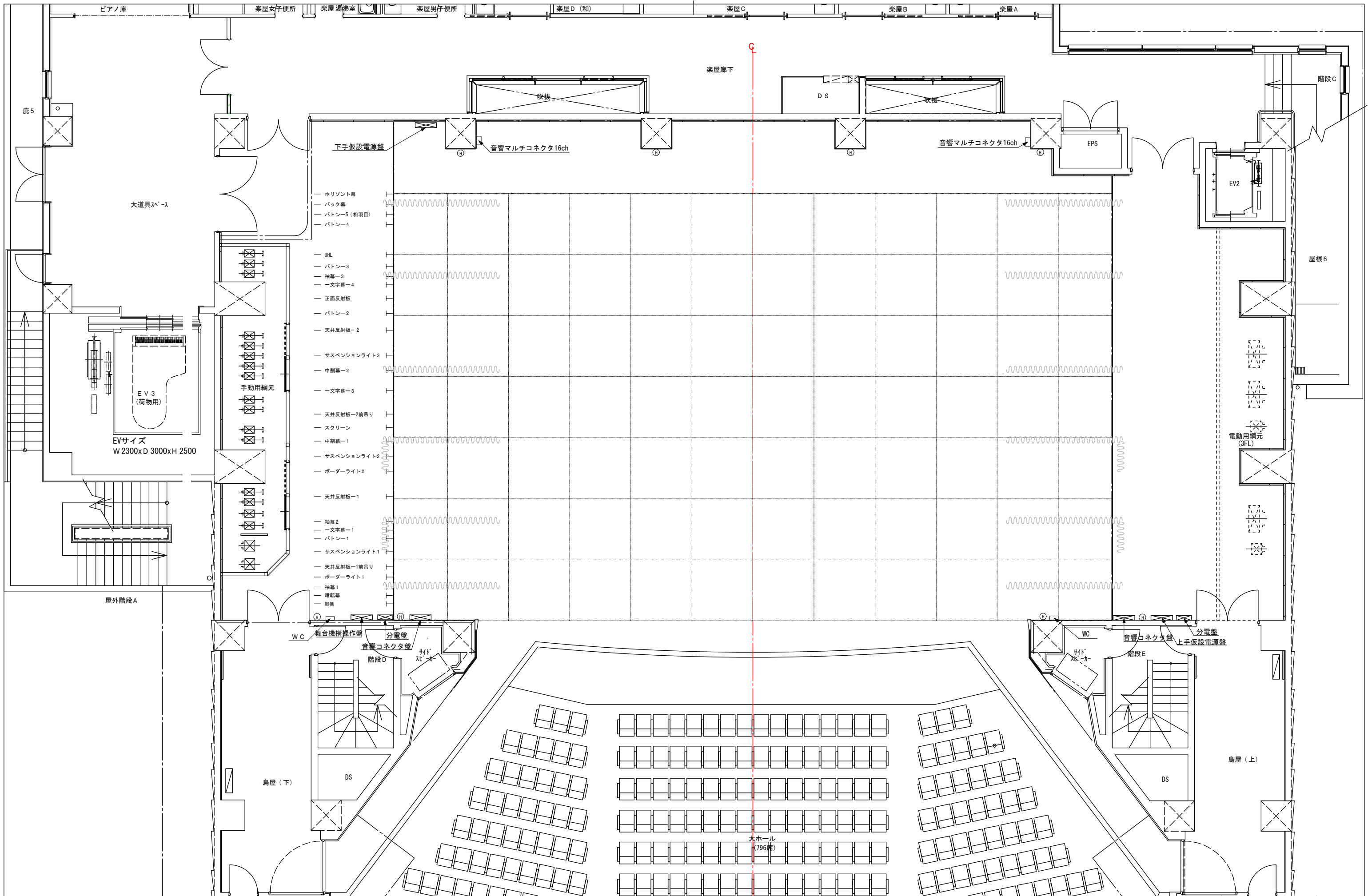
おりなす八女 ハーモニーホール 平面図
